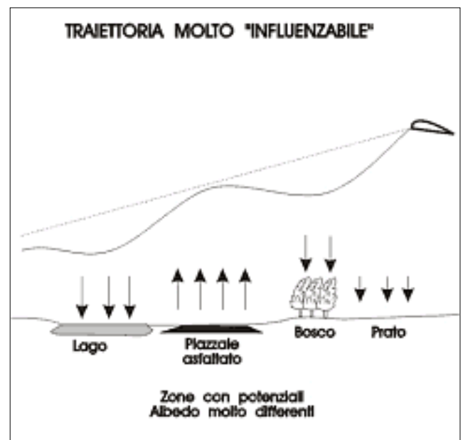
Figura 8-18. Sorvolando terreni con caratteristiche termiche differenti la traiettoria di discesa può venire notevolmente influenzata.
