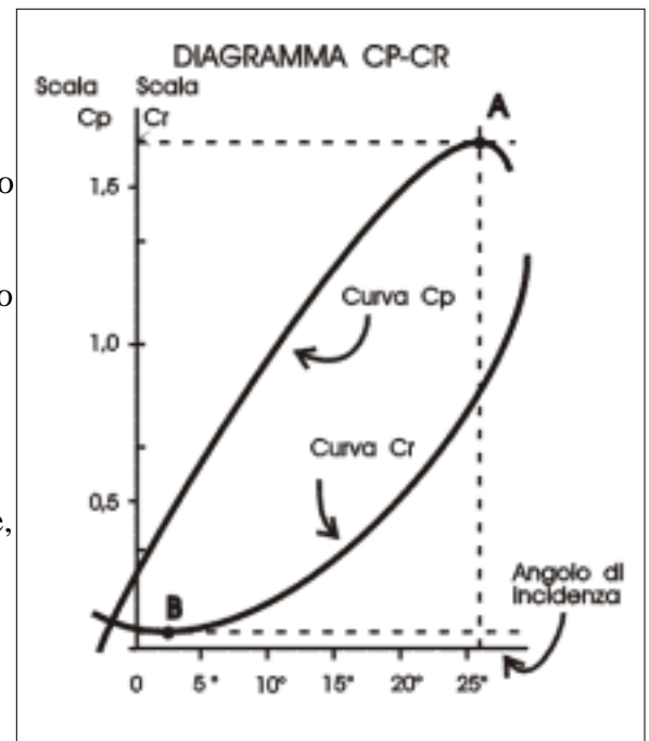
Figura 3-16. Diagramma Cp-Cr.
