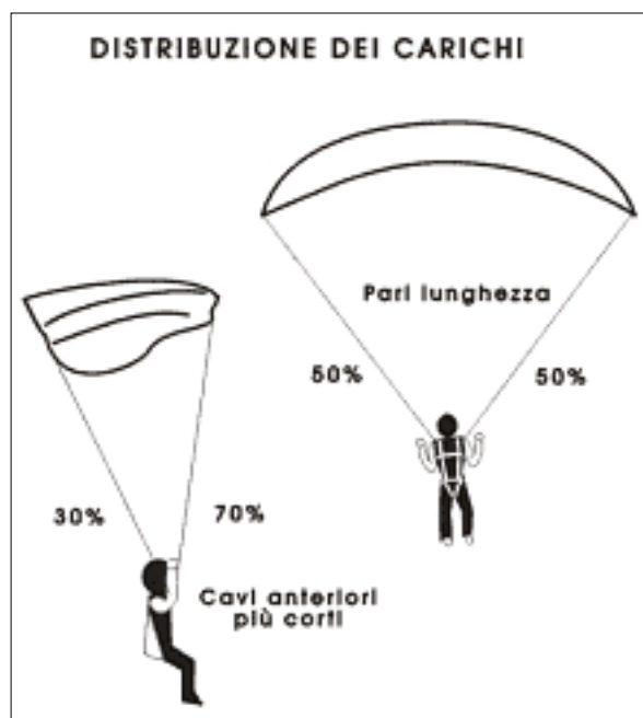
Figura 6-24. La distribuzione dei carichi dipende direttamente dalla lunghezza dei cordini.
