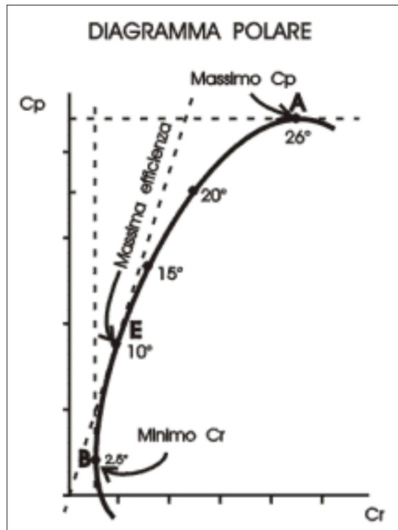
Figura 3-17. Diagramma Polare.
