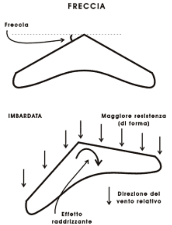
Figura 5-36. L'angolo di freccia conferisce stabilità rotatoria generando differenze di resistenza.
