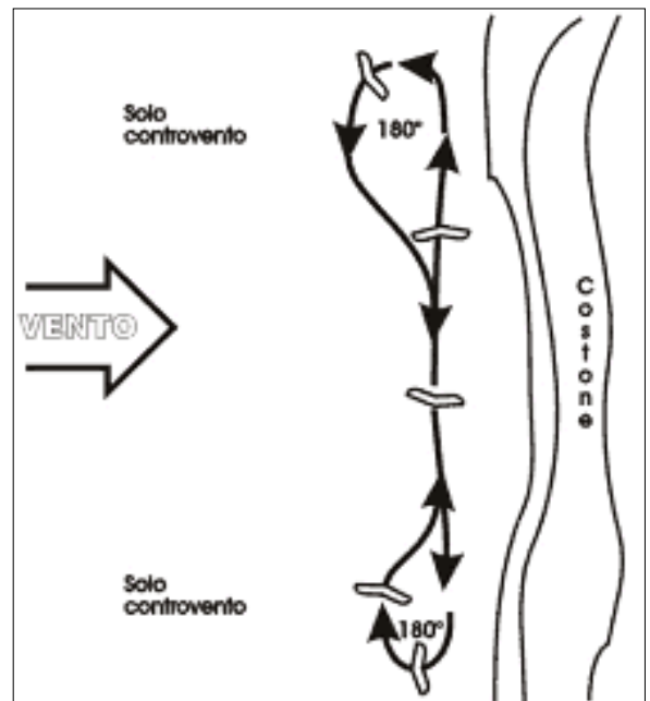
Figura 8-9. Volare in dinamica significa "bordeggiare" il pendio mantenendosi sempre alla giusta distanza da questo e compiendo le virate sempre controvento.
