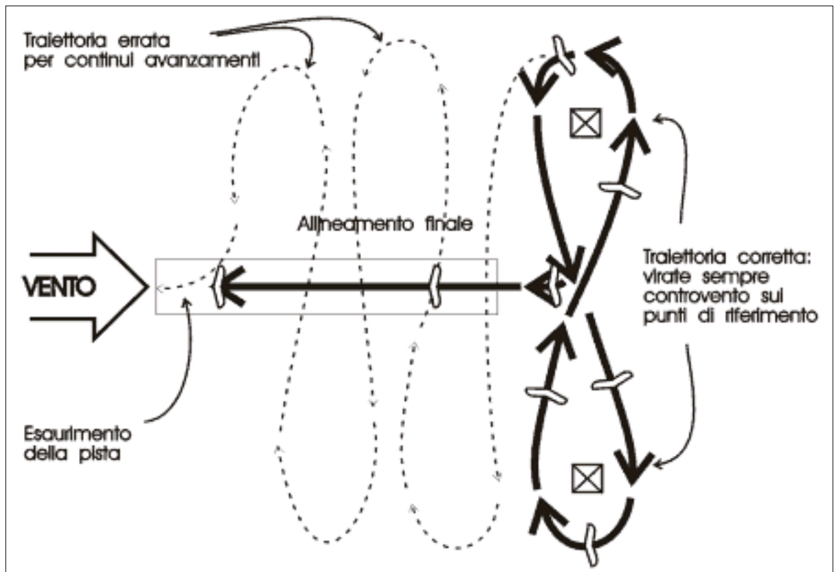
Figura 2-4. Circuito ad 8: i riferimenti al suolo verranno presi considerando l'efficienza del mezzo (deltaplani più arretrati, parapendio più vicini all'inizio della pista) e l'intensità del vento (tanto più avanzati quanto maggiore è il vento); la assenza
