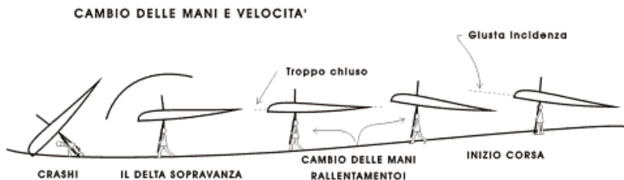
Figura 5-15. L'errato (ed involontario) rallentamento al momento del cambio delle mani, determina una accelerazione del deltaplano che ci sopravanza: è necessario evitare il rallentamento e mantenere la progressiva della corsa.
