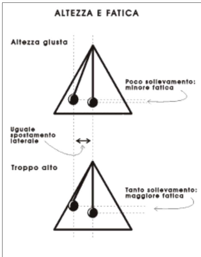
Figura 5-9. Un aggancio troppo alto richiede un maggior sforzo per ottenere lo stesso spostamento laterale del peso
