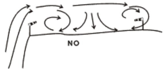
Figura 5-19. Gli alberi in fondo limitano lo spazio utile per il decollo. Gli strapiombi devono essere assolutamente evitati
