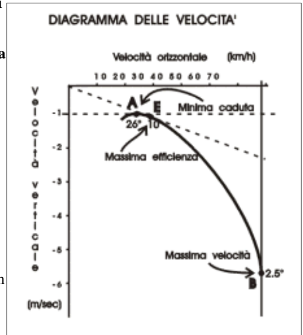
Figura 3-18. Diagramma delle Velocità.
