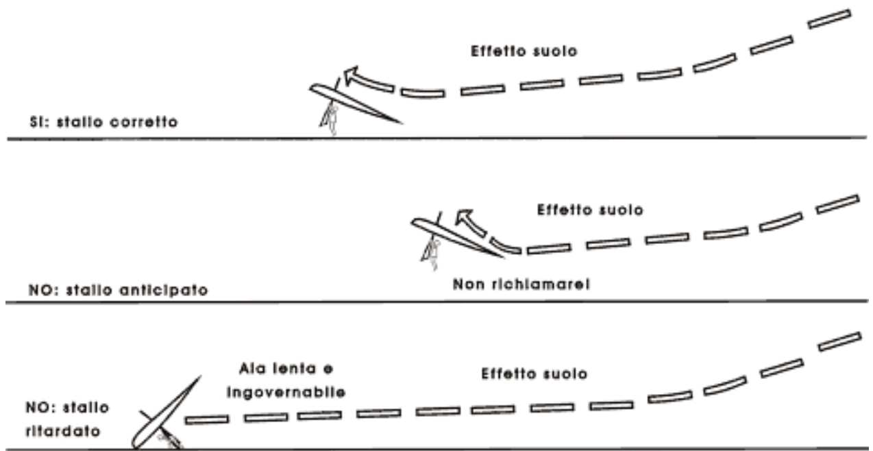
Figura 5-16. Stallando troppo presto il delta si rialza, ritardando esso non si ferma, ma spaccia fino al suolo.
