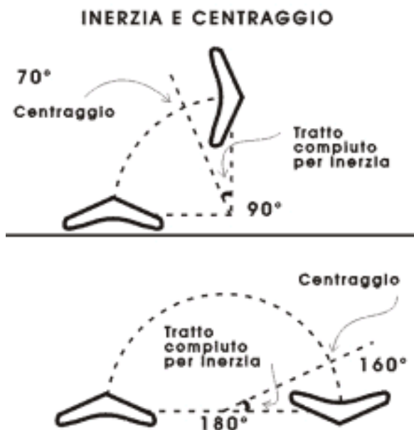
Figura 5-22. L'inerzia dell'apparecchio richiede che il "centraggio" venga effettuato in anticipo (20° < 180° circa).
