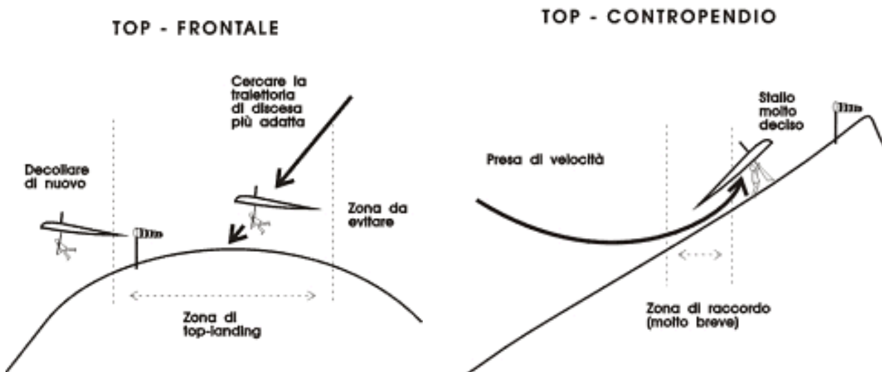
Figura 5-29. Top landing con vento frontale: è possibile solo in alcune zone particolarmente favorevoli.
