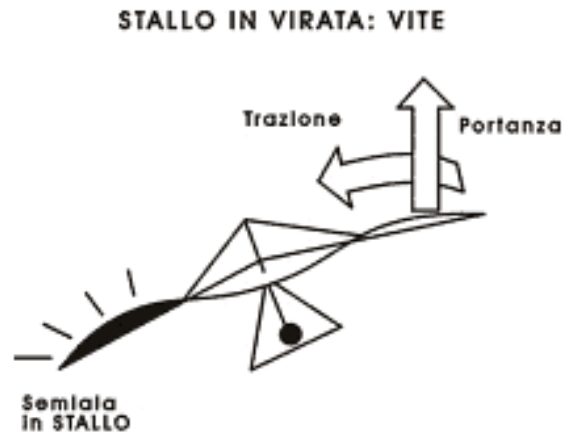
Figura 5-25. Stallo d'ala (vite) per scarsa velocità in entrata od eccessiva cabrata.
