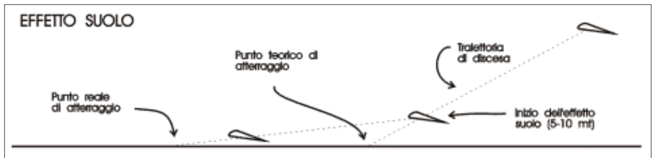
Figura 3-23. L'effetto suolo "allunga" notevolmente la traiettoria finale durante l'atterraggio
