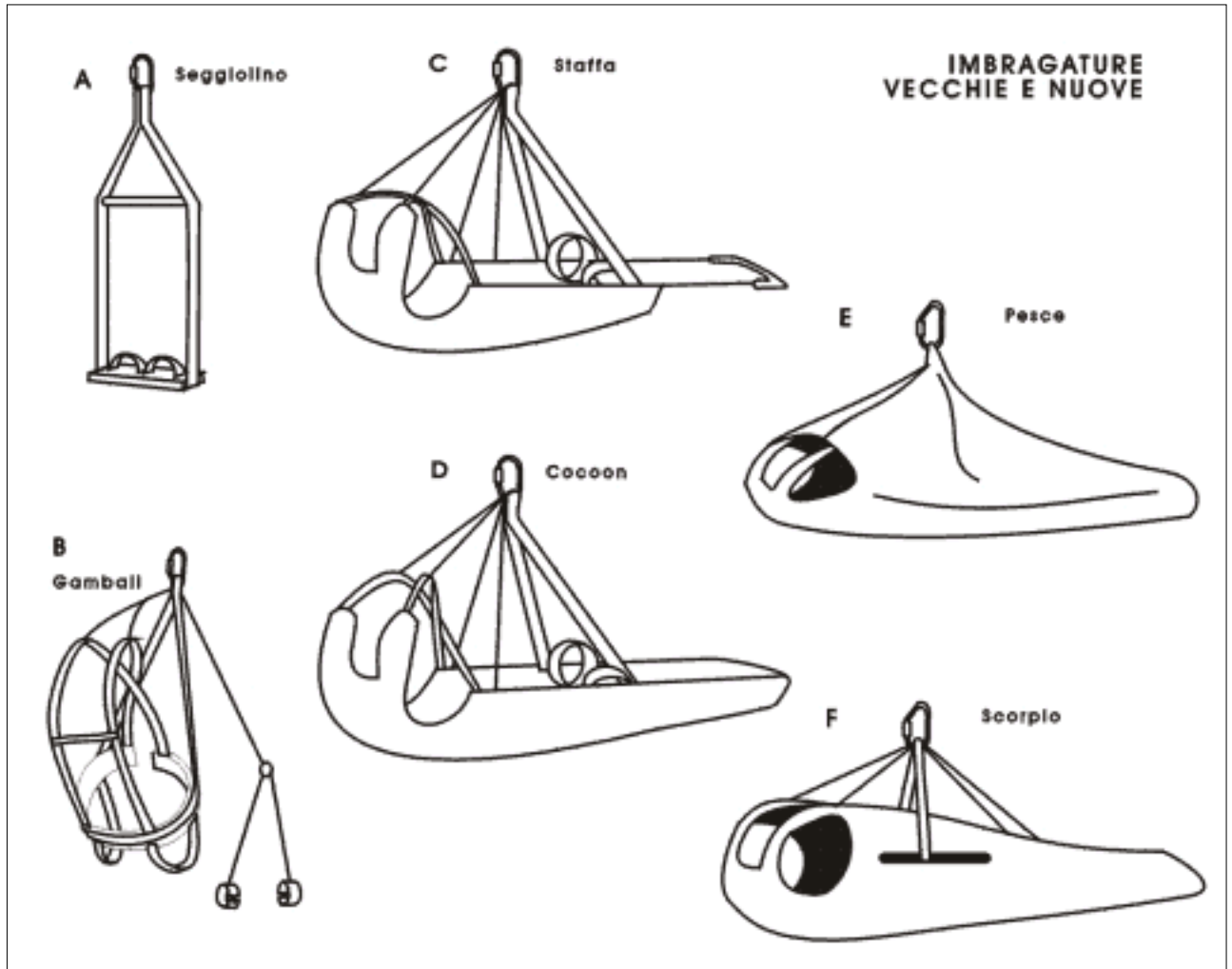
Figura 5-7. Modelli di imbragatura
