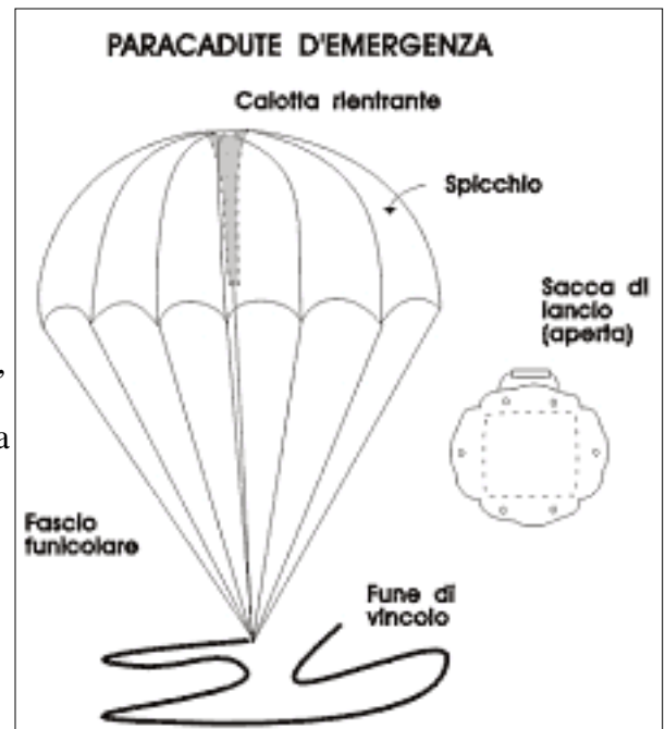
Figura 7-1. Il paracadute d'emergenza per il volo libero.
