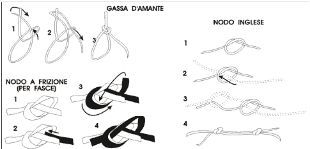
Figura 7-6. Tre nodi da imparare e ricordare
