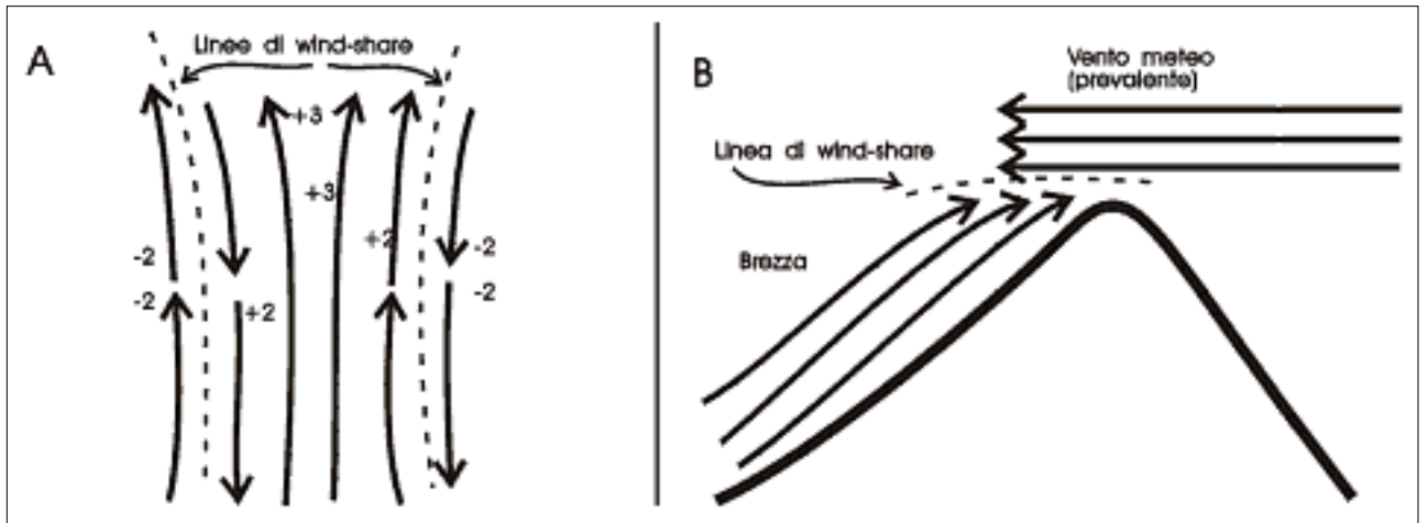
Figura 4-20. A: Wind-share verticale (ai margini di una termica) . B: wind-share orizzontale (formato dalla brezza e dal vento prevalente).
