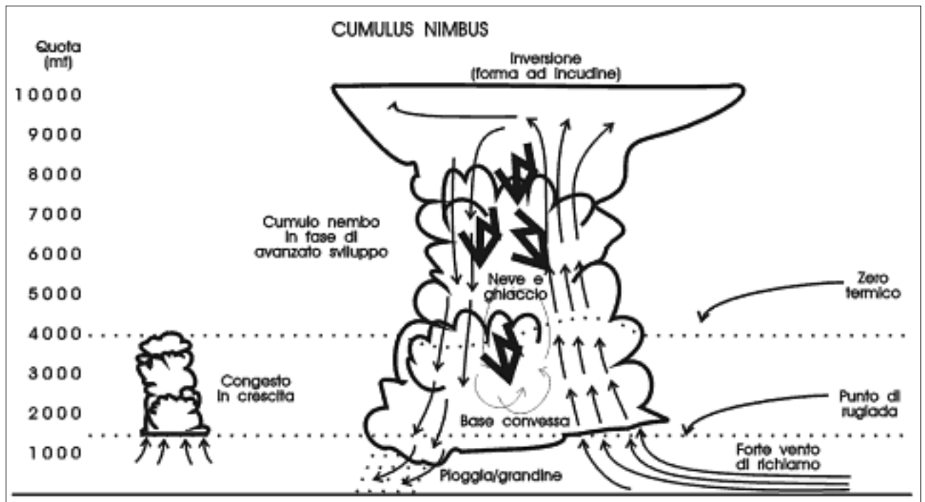
Figura 4-23. Linee di flusso d'aria e dimensioni relative di un Cumulus nimbos: per la forza dei venti ad esso associati e per la notevole turbolenza creata, questa nube viene evitata anche dai grandi aerei di linea.
