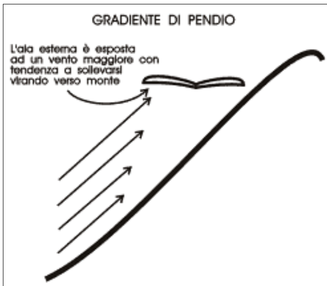
Figura 4-19. Gradiente di vento sul pendio.
