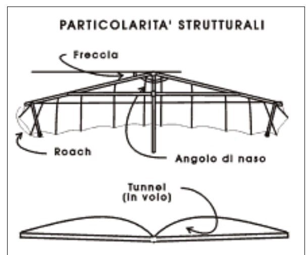
Figura 5-3. Angolo di naso, freccia a roach
