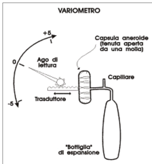
Figura 7-4. Il variometro, un misuratore delle variazioni istantanee di pressione.
