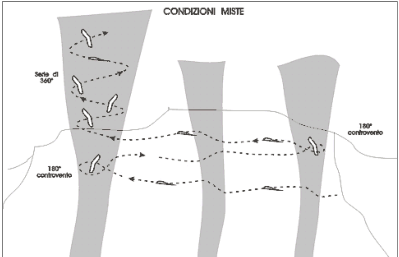
Figura 8-13. Sfruttamento delle ascendenze "miste": a bassa quota si compie una serie di 180° e, superata abbondantemente la linea di cresta, si iniziano i 360° nella termica più potente individuata.
