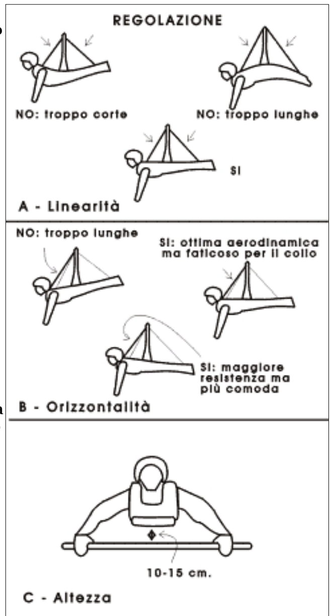
Figura 5-8. Le tre fasi della regolazione di un'imbragatura: linearità, orizzontalità e distanza dalla
