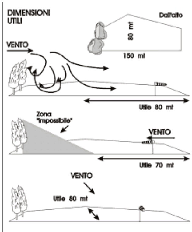
Figura 8-15. Influenza della direzione del vento sulle dimensioni realmente sfruttabili di un campi di atterraggio.
