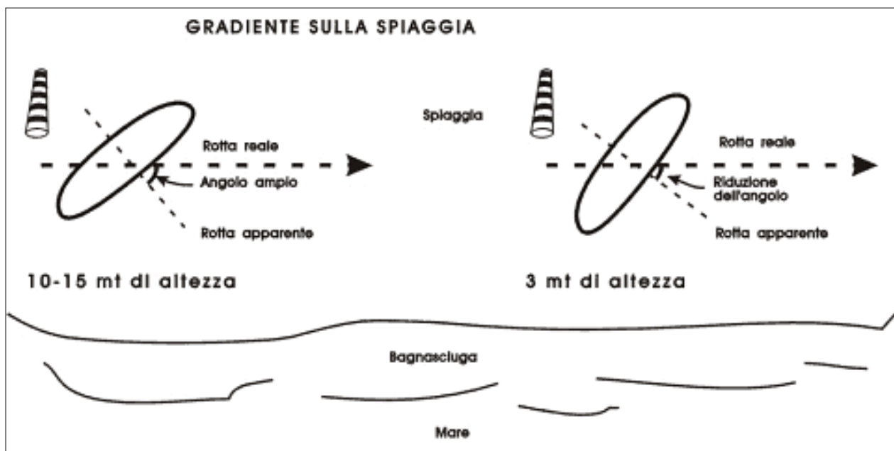
Figura 6-23. Il gradiente di vento su una spiaggia ha il perverso effetto di "attirare" la vela verso l'acqua: per evitare ciò si deve ridurre l'angolo di deriva man mano che ci si avvicina al suolo.
