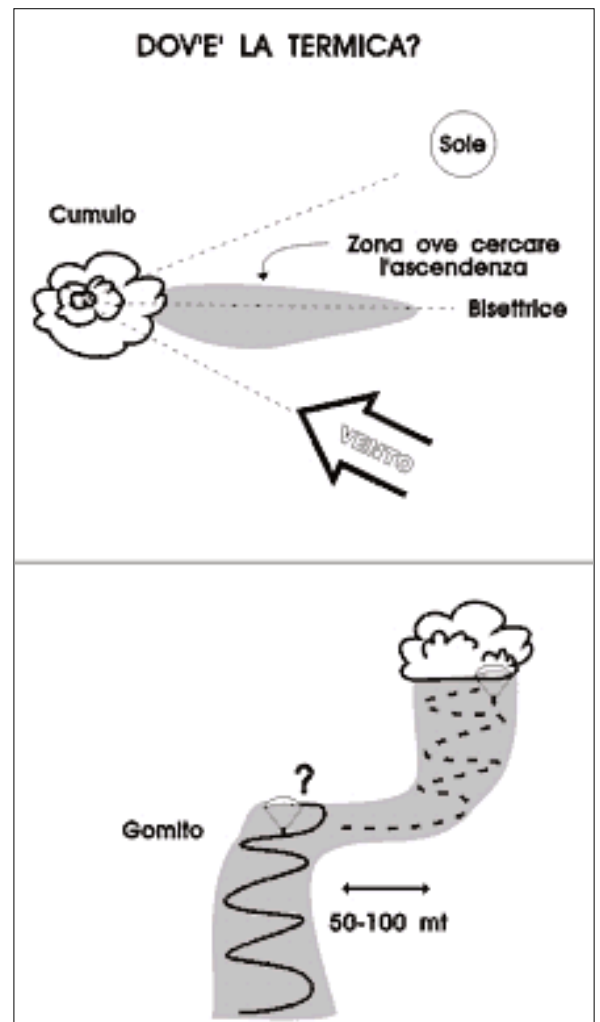
Figura 8-5. La zona di ascendenza deve essere ricercata sulla bisettrice dell'angolo che il cumulo forma con il sole e con la direzione del vento. A volte le termiche formano veri e propri gomiti, e proseguono sottovento.
