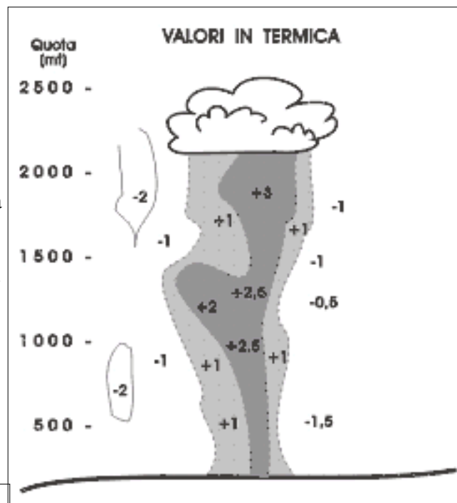
Figura 8-1. Una termica reale: si noti la zona centrale di maggiore ascendenza e la irregolarità della forma.
