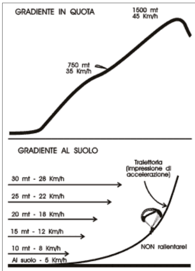
Figura 4-18. Gradienti di vento in quota ed al suolo.
