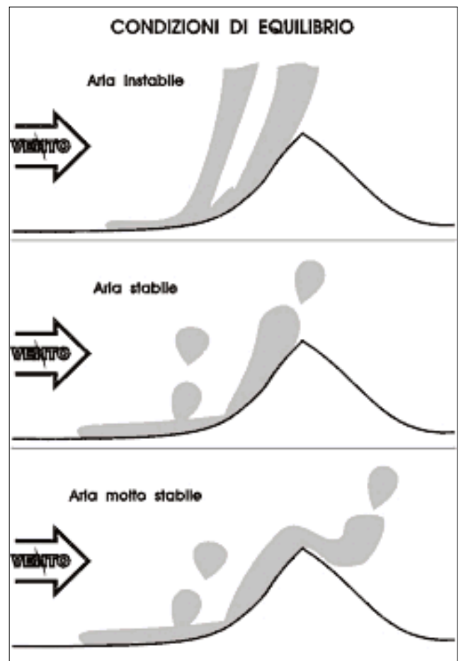
Figura 8-3. Naturalmente la stabilità dell'aria è determinante: aria instabile=termiche frequenti e che raggiungono quote elevate.
