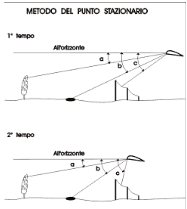
Figura 8-17 Trigonometria del punto stazionario (spiegazioni nel testo).
